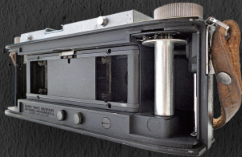
»Stereo Realist« Rückseite Negativformat 23,1 x 25,4 mm
